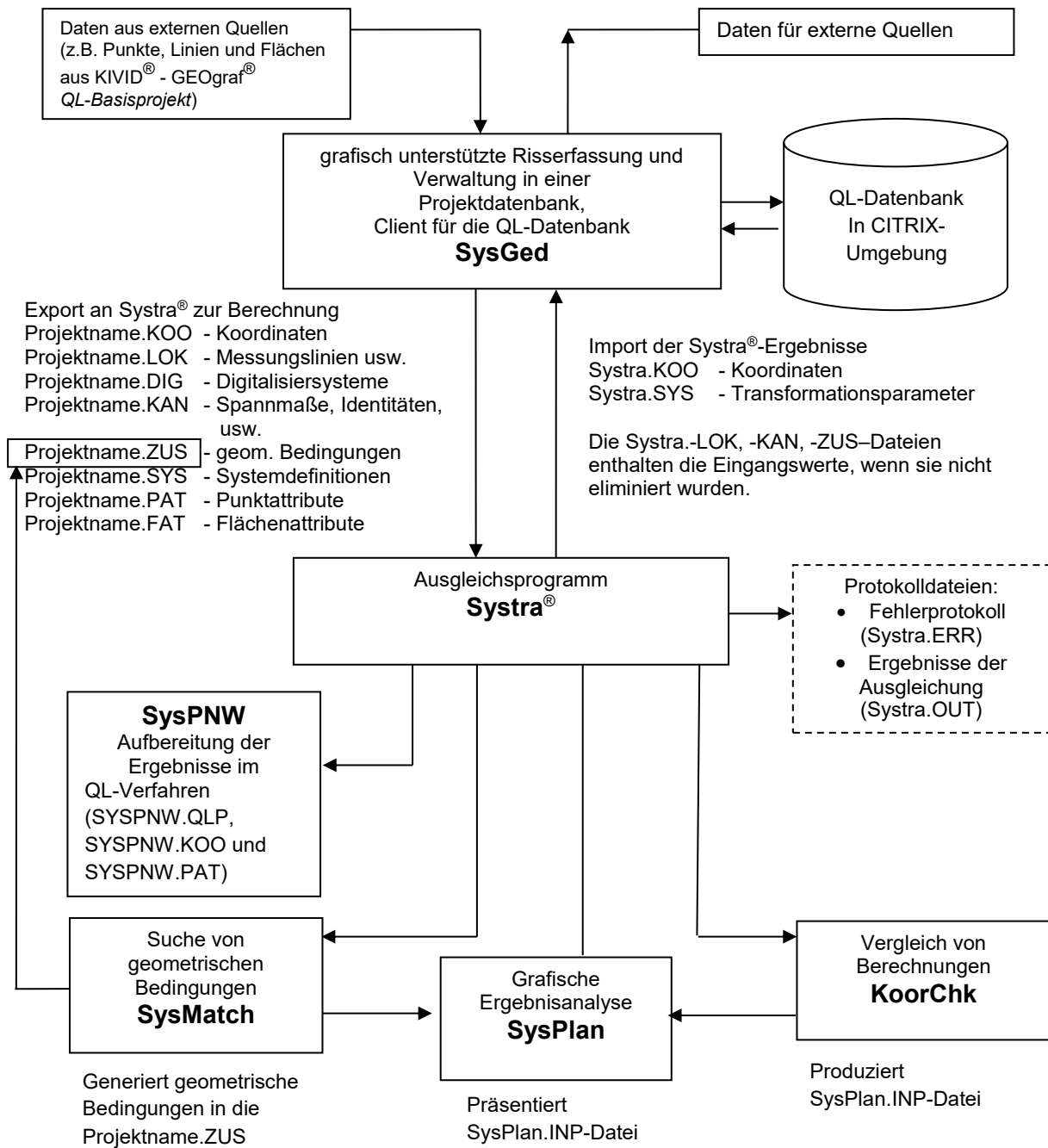
Übersicht 2: Datenfluss im Programmsystem Systra®
