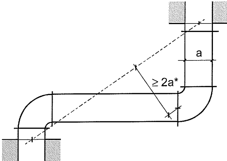
Bild 5.1: Begrenzung der Kraffteinleitung mit Leitungsverziehung
