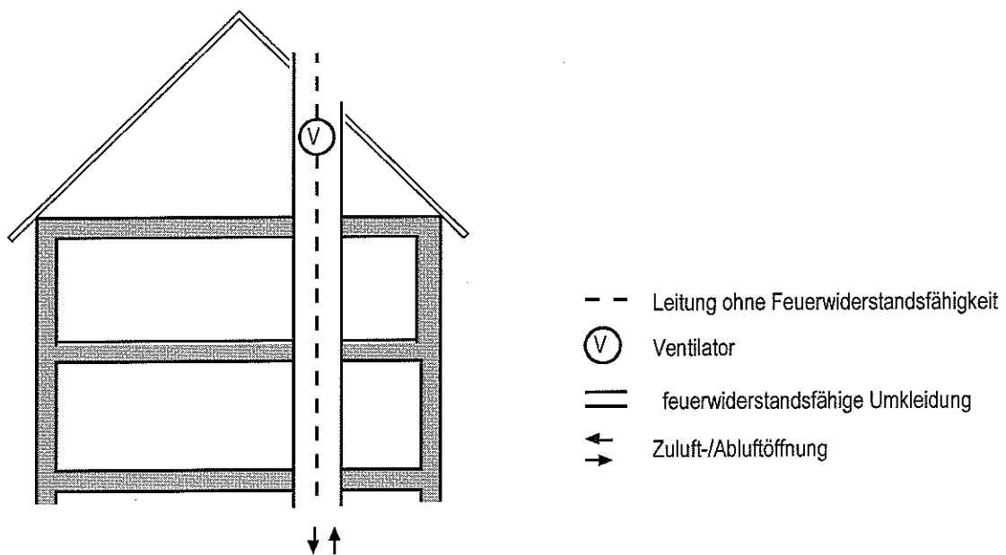
Bild 2.2: Schachtlösung
