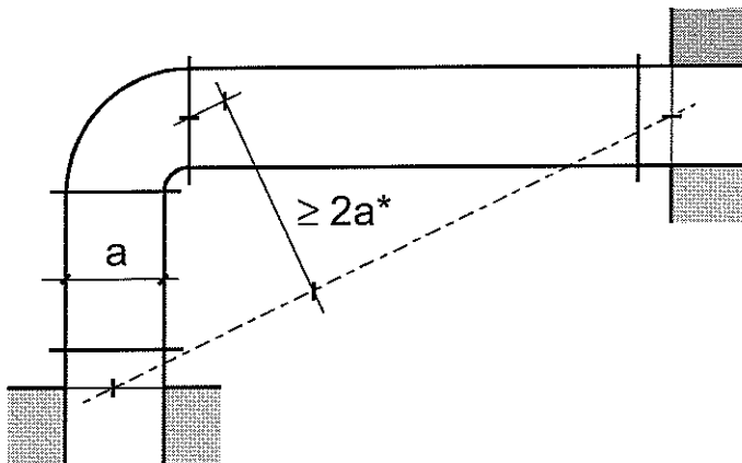
Bild 5.2: Begrenzung der Kraffteinleitung mit Bogen
