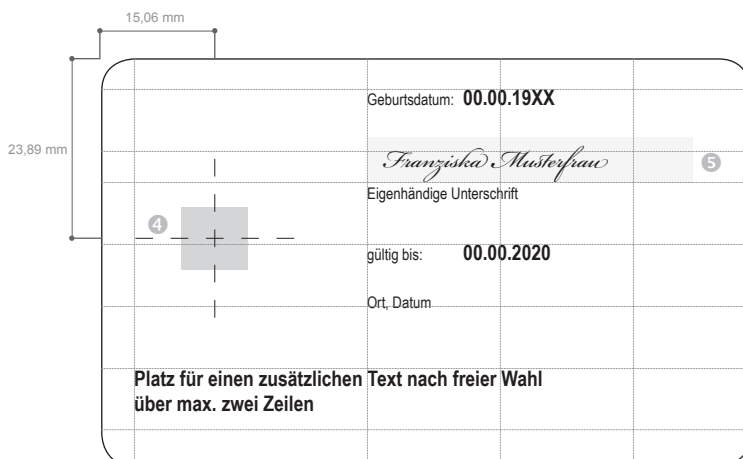
Ansicht Rückseite 100 %
